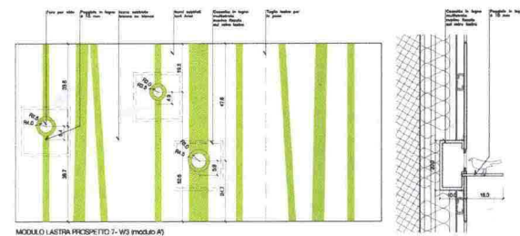
MODULO LASTRA PROSPETTO 1-VIS (modulo A)
